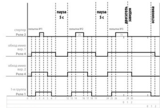
Типовая Диаграмма. Тип 1 Диаграмма запуска двигателя для автомобилей концерна VAG с традиционным замком зажигания, а также для автомобилей Mercedes и BMW с использованием модуля A3/D3 типа Fortin)
